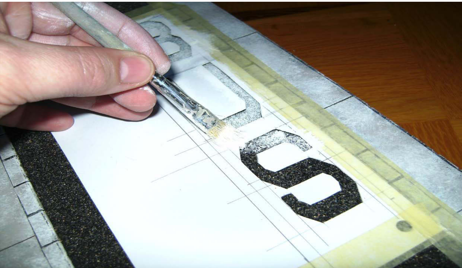
Auftupfen des Schriftzuges „BUS“
